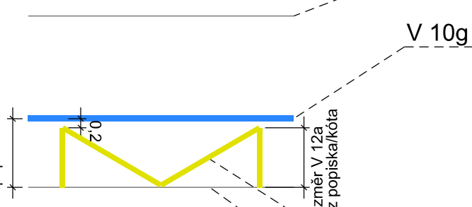
Vzorový vzhled instalovaného značení V 12a
