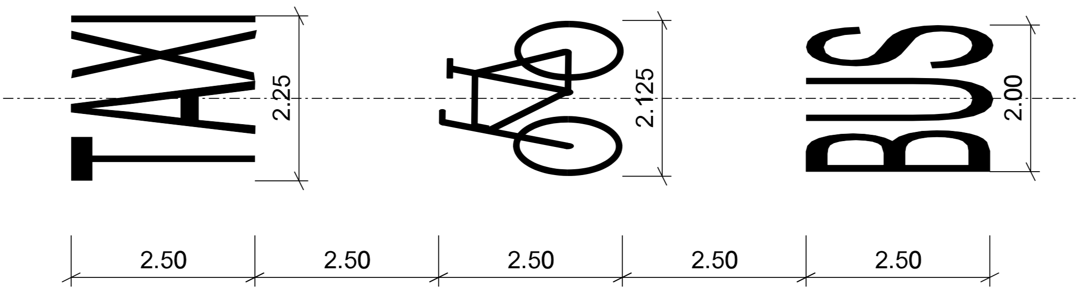
VZOR VODOROVNÉHO DZ č. V 15:
